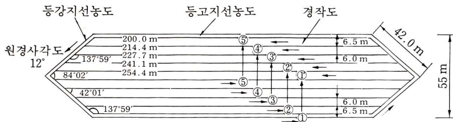
(a) 귀갑형 도로배치
