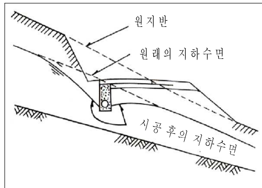
그림 4.5.5 차단배수구의 예
