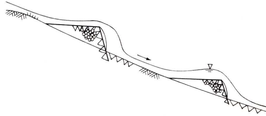
그림 4.1.26 자연배수대의 소낙차공
