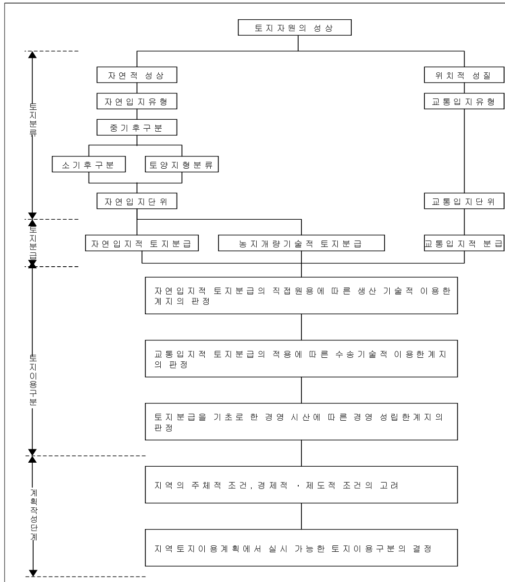
그림 3.2.1 토지이용구분방법의 개념도
