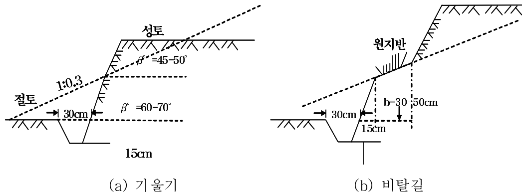
그림 4.1.14 계단 비탈면
