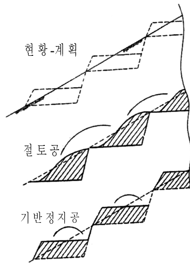
그림 4.1.9 전단면 절토공법
