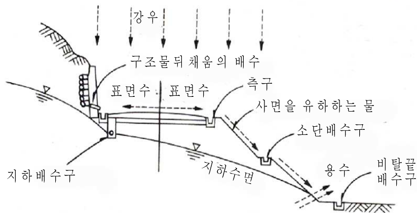
그림 4.5.3 농도의 배수처리
