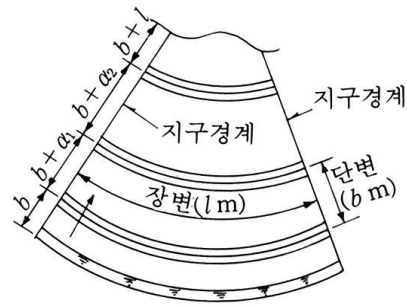
그림 4.1.12 전단면 절토공 평면도
