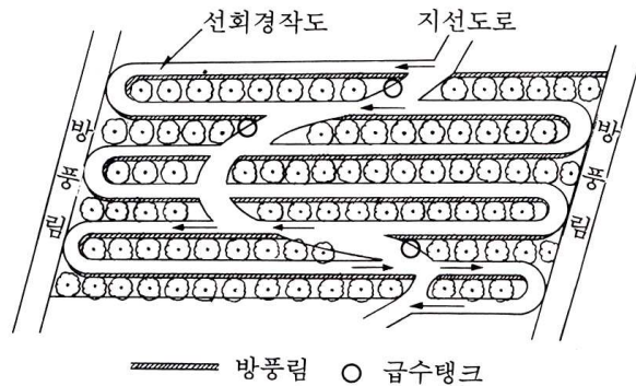
그림 4.1.21 양단선회식 농도배치
