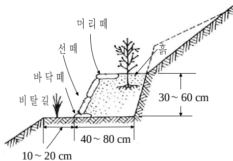
그림 4.6.3 선폐공
