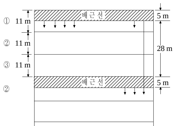
그림 4.1.6 배근거리와 배근선
