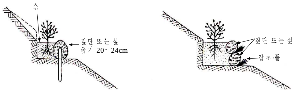
그림 4.6.2 짚단·싹 덮기
