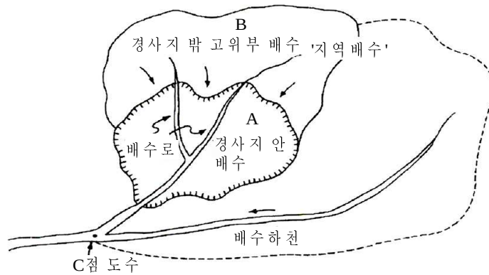
그림 4.4.3 배수구역 개념도
