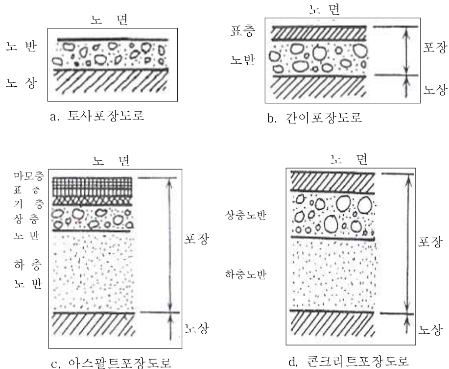
그림 4.5.2 도로의 구조 분류
