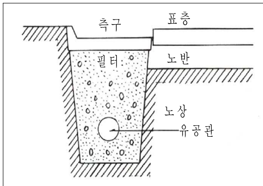
그림 4.5.4 노반 및 노상배수구의 예
