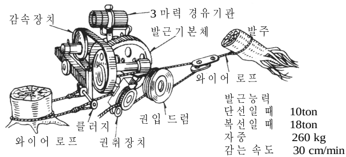
그림 4.1.1 원치 뿌리뽑기
