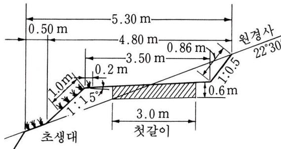
그림 4.1.10 계단공의 토공량 계산 예
