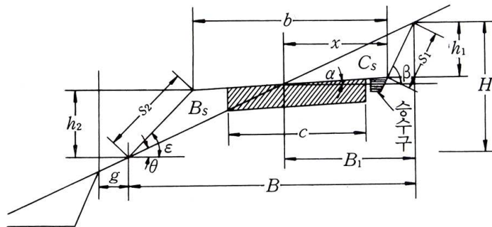
그림 4.1.13 계단밭의 표준단면
