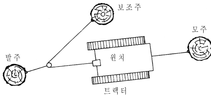
그림 4.1.4 트랙터 윈치에 의한 뿌리뽑기
