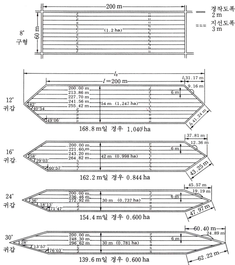
그림 4.1.20 원경사도에 대응한 경작도 배치
