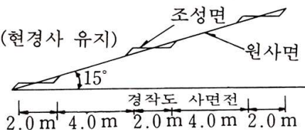
그림 4.1.16 경작도형 사면전의 표준단면도
