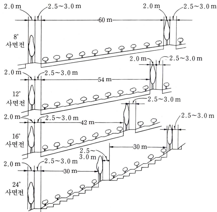
그림 4.1.19 원경사도별 사면전 횡단배치도
