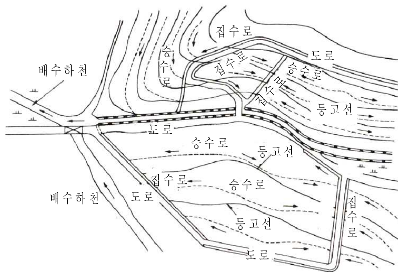
그림 4.4.5 배수로의 배치(예)
