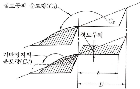
그림 4.1.11 절토와 정지 운반토량
