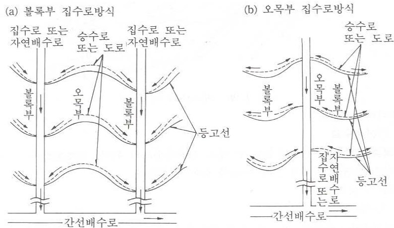
그림 4.4.4 집수로의 배치계획(예)
