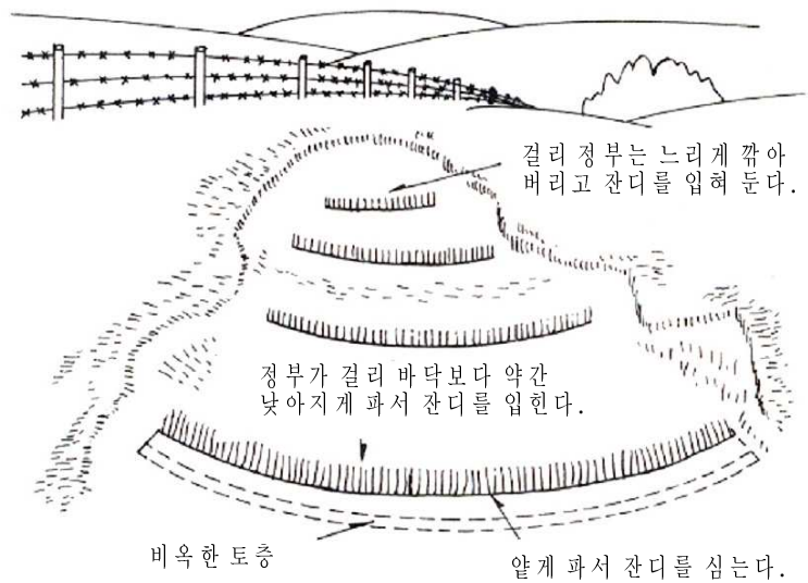
그림 4.6.7 잔디 저지보
