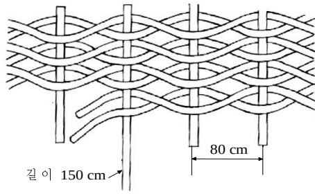
그림 4.6.5 편책공
