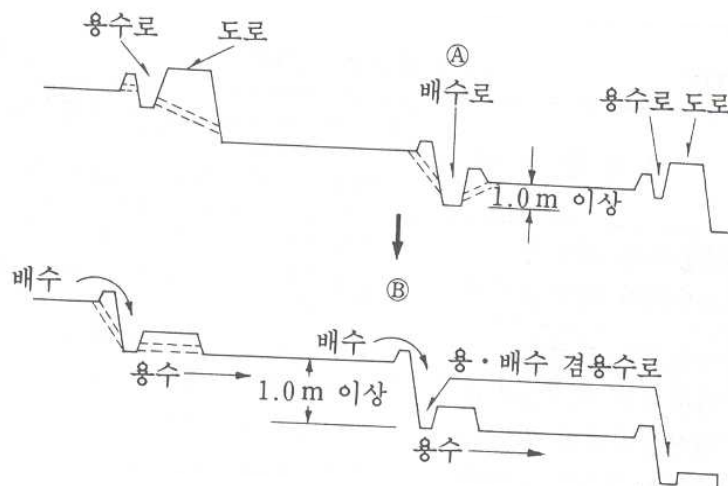
그림 4.5.1 농도와 용·배수로의 관계
