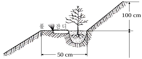
그림 4.6.6 플계단공
