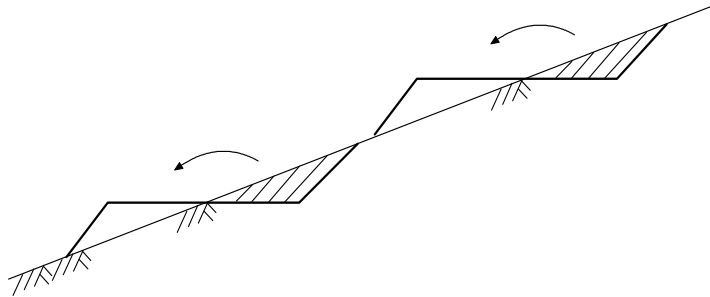
그림 4.1.8 절·성토공법
