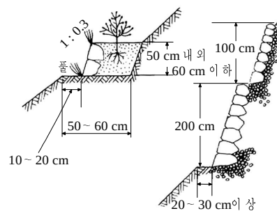
그림 4.6.4 석축공
